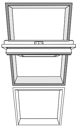
Oben Zweiteiliges Dachfenster Maßunterschiede beachten zwischen Typ 1 und Typ 2
